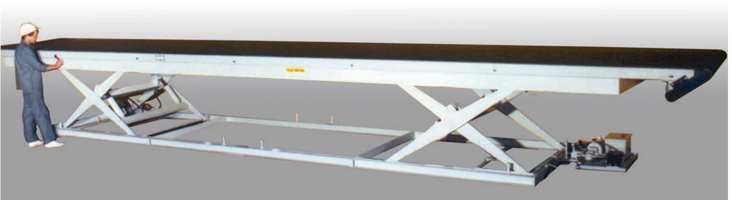
Groß-Förderband mit integrierter Tandem-Scherenhebebühne Large belt conveyor mounted on a tandem scissor lift
